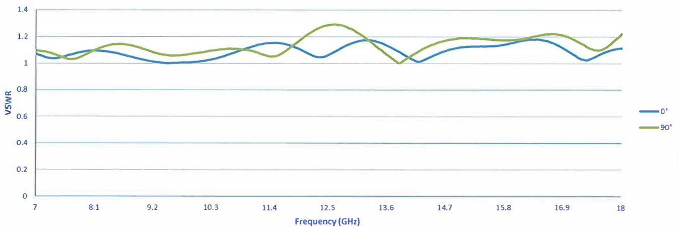
VSWR
