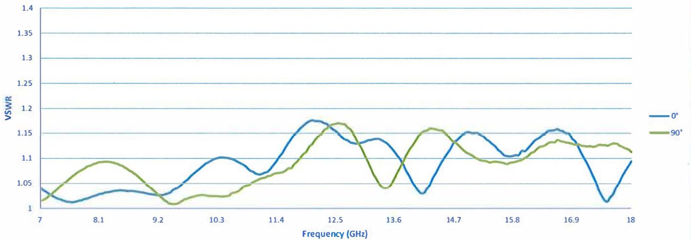
VSWR
