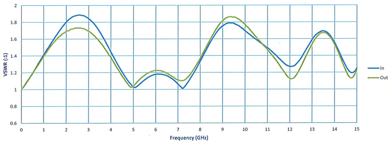
VSWR
