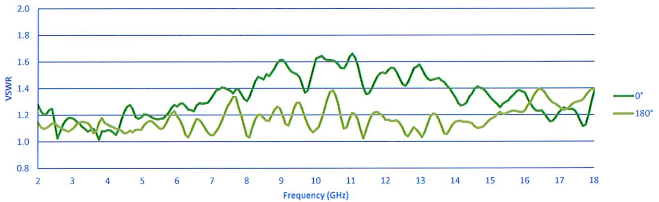
VSWR (Input)
