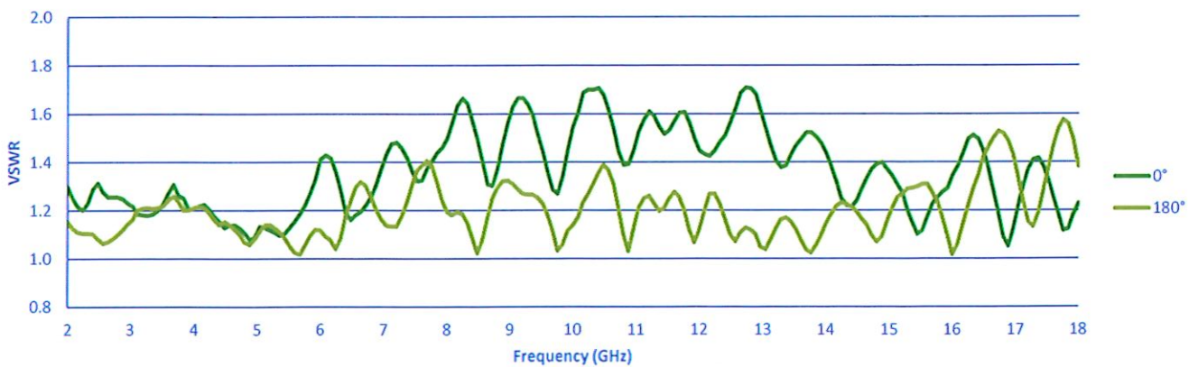
VSWR (Output)
