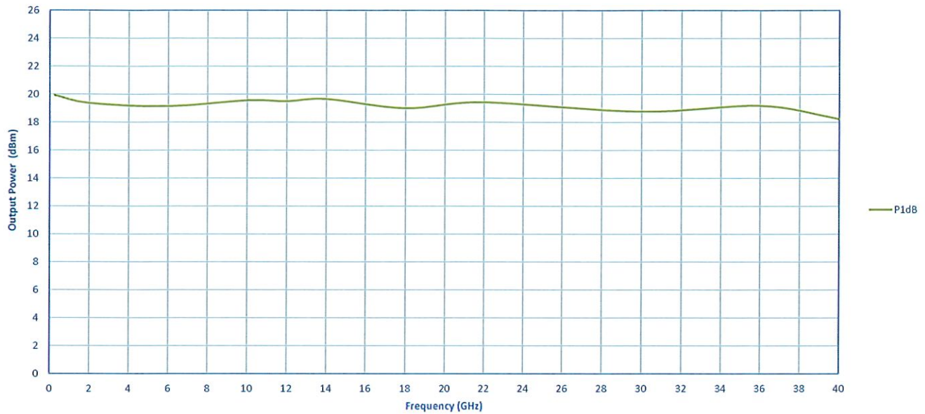
OP1dB
