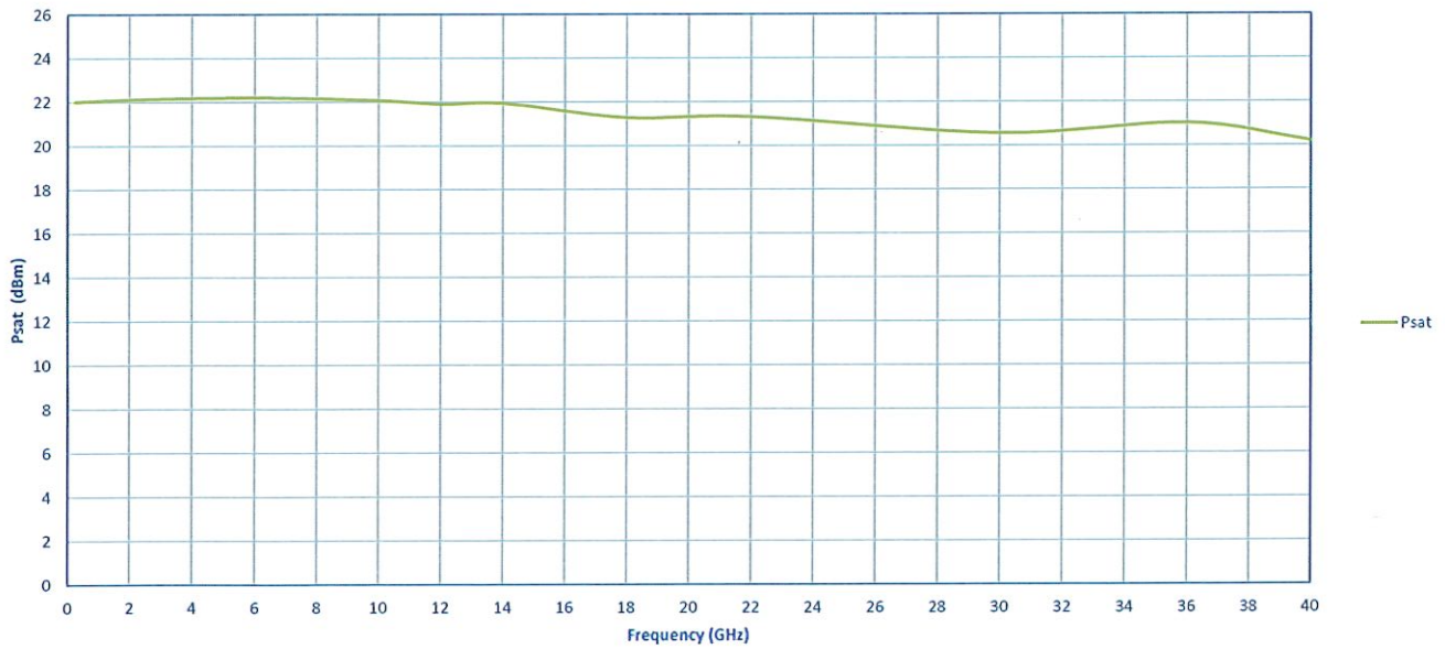
PSAT
