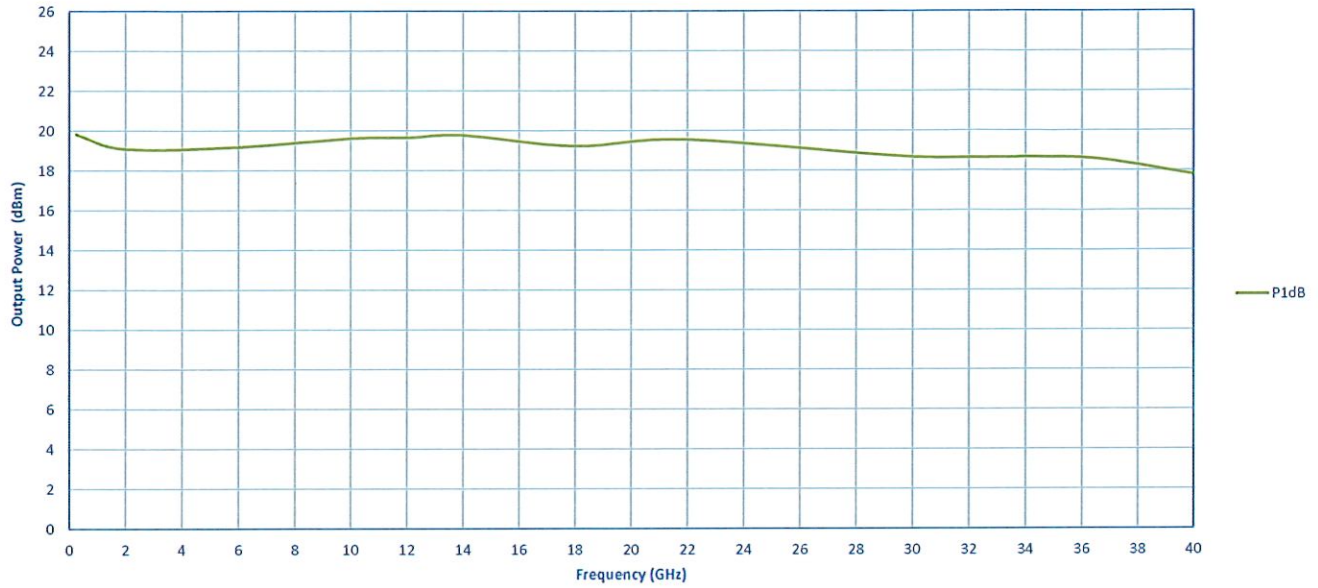
OP1dB
