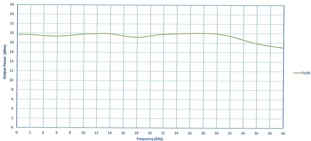
OP1dB
