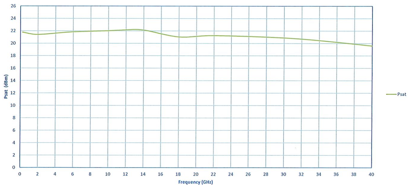
PSAT
