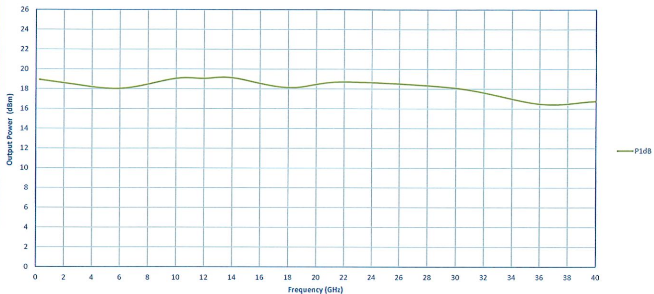
OP1dB
