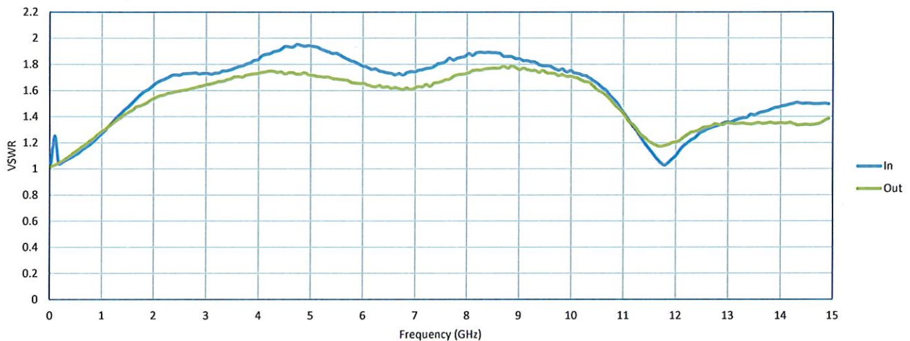
VSWR
