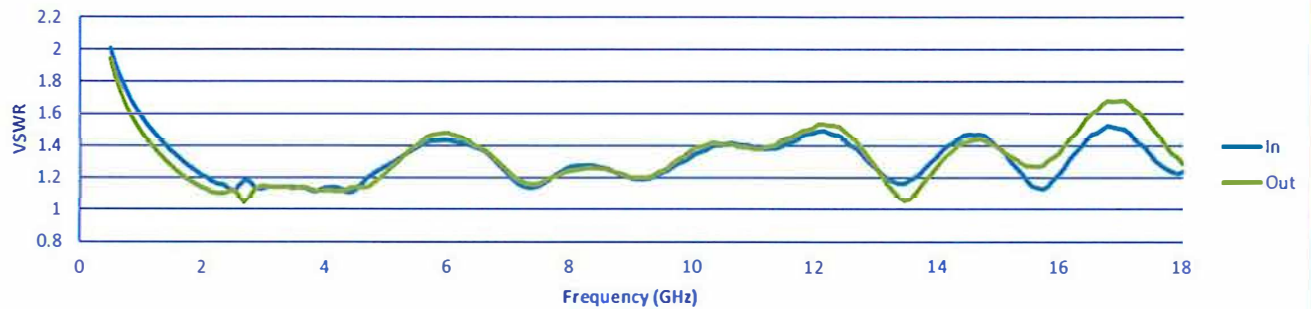
VSWR
