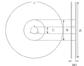
Reel Dimensions
