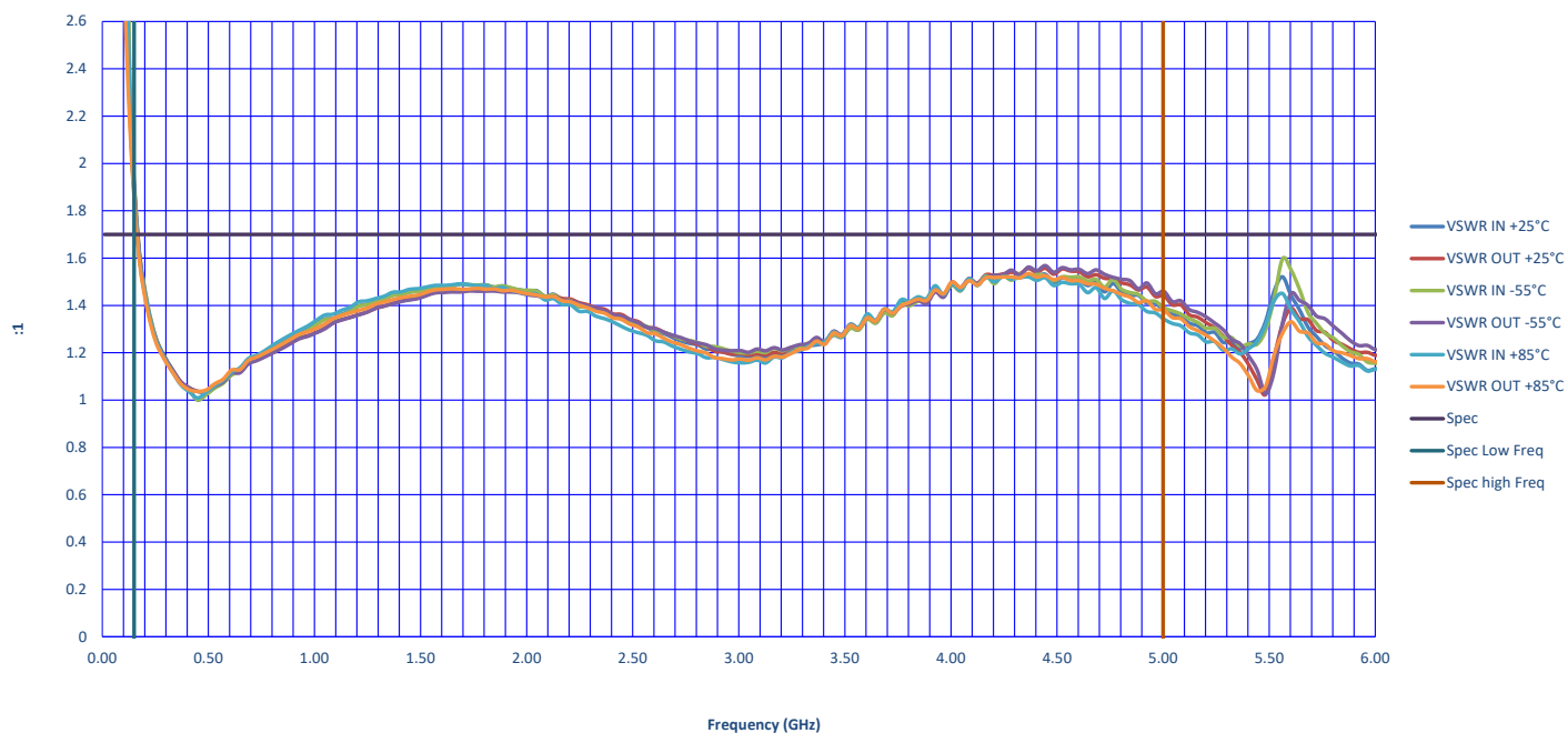
VSWR
