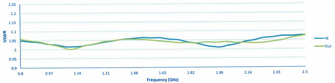
VSWR
