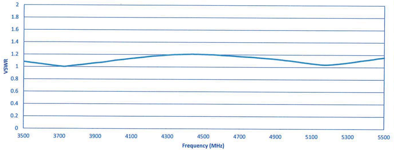
VSWR
