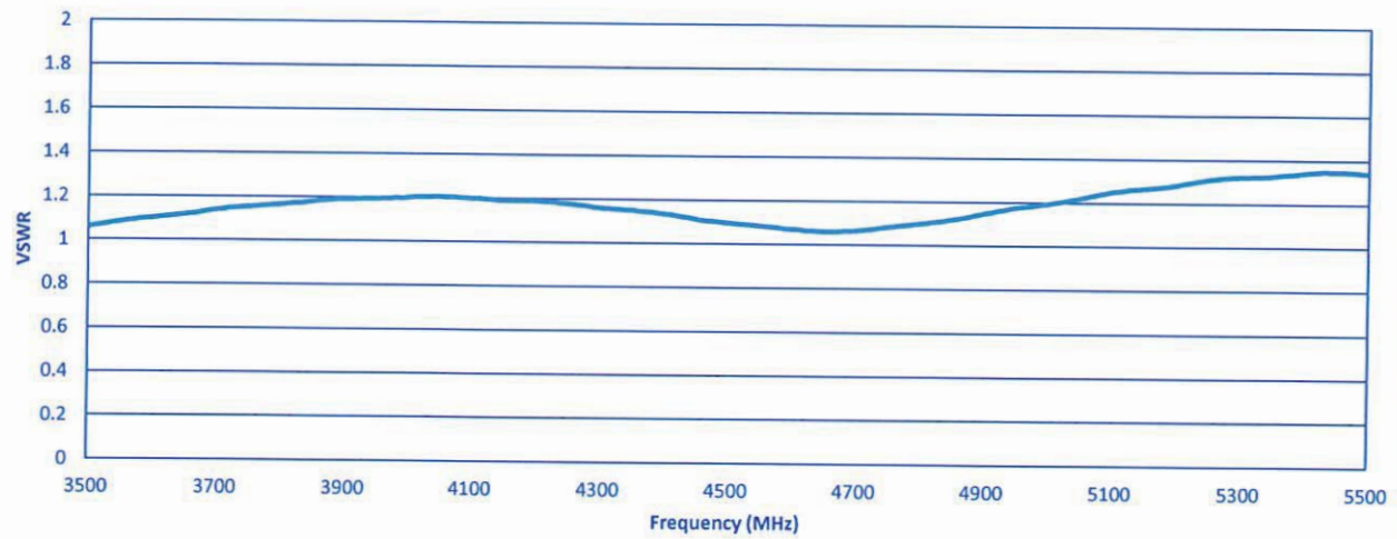
VSWR
