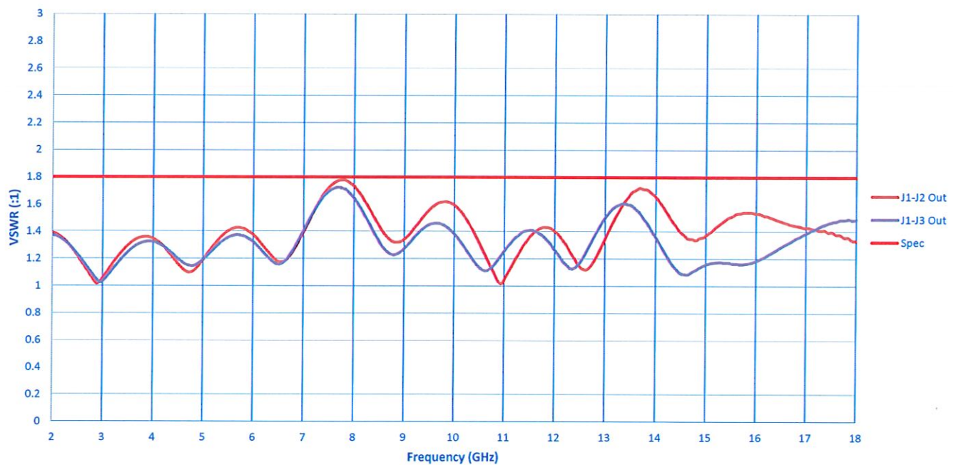
VSWR (Out)
