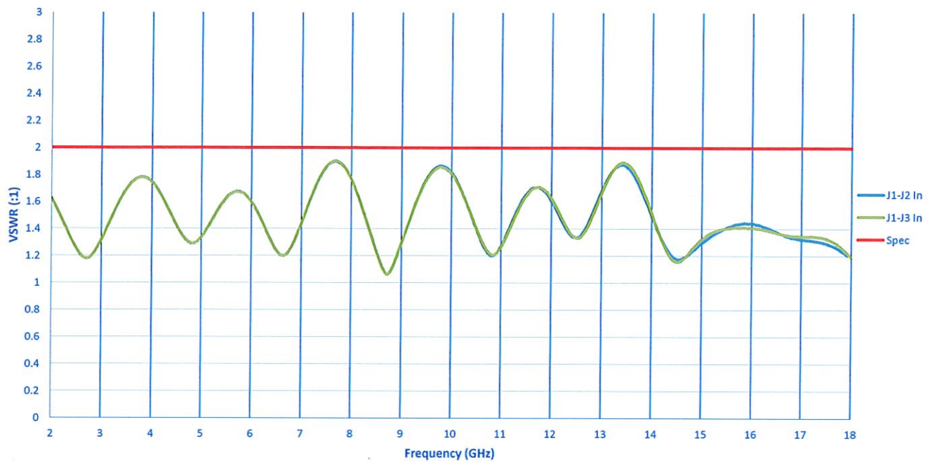
VSWR (In)
