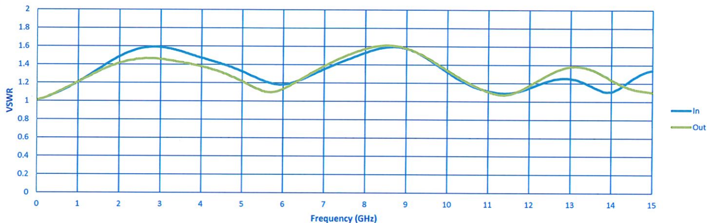
VSWR
