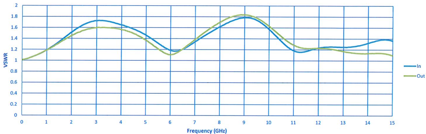
VSWR
