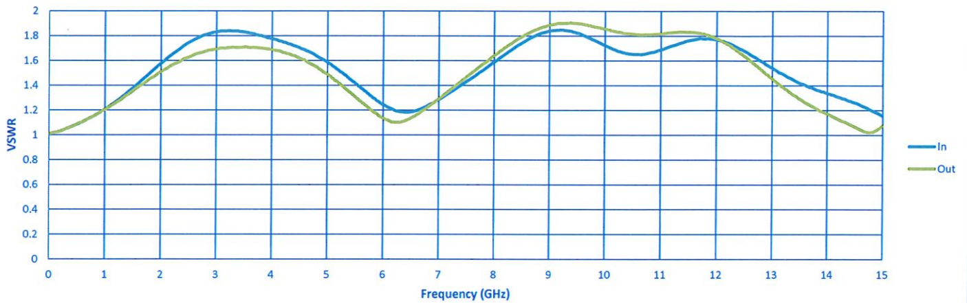
VSWR
