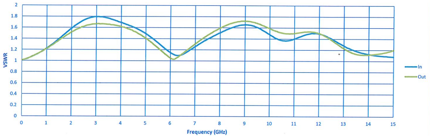
VSWR
