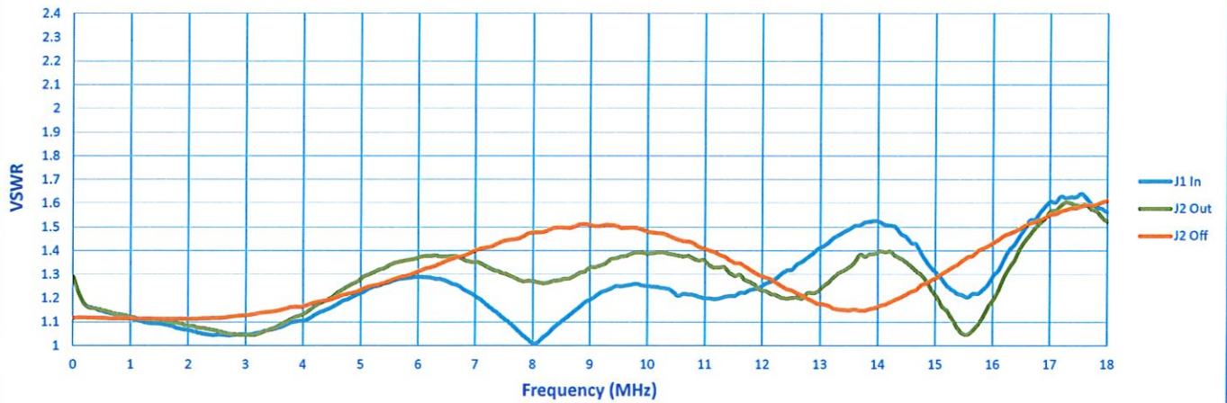
VSWR
