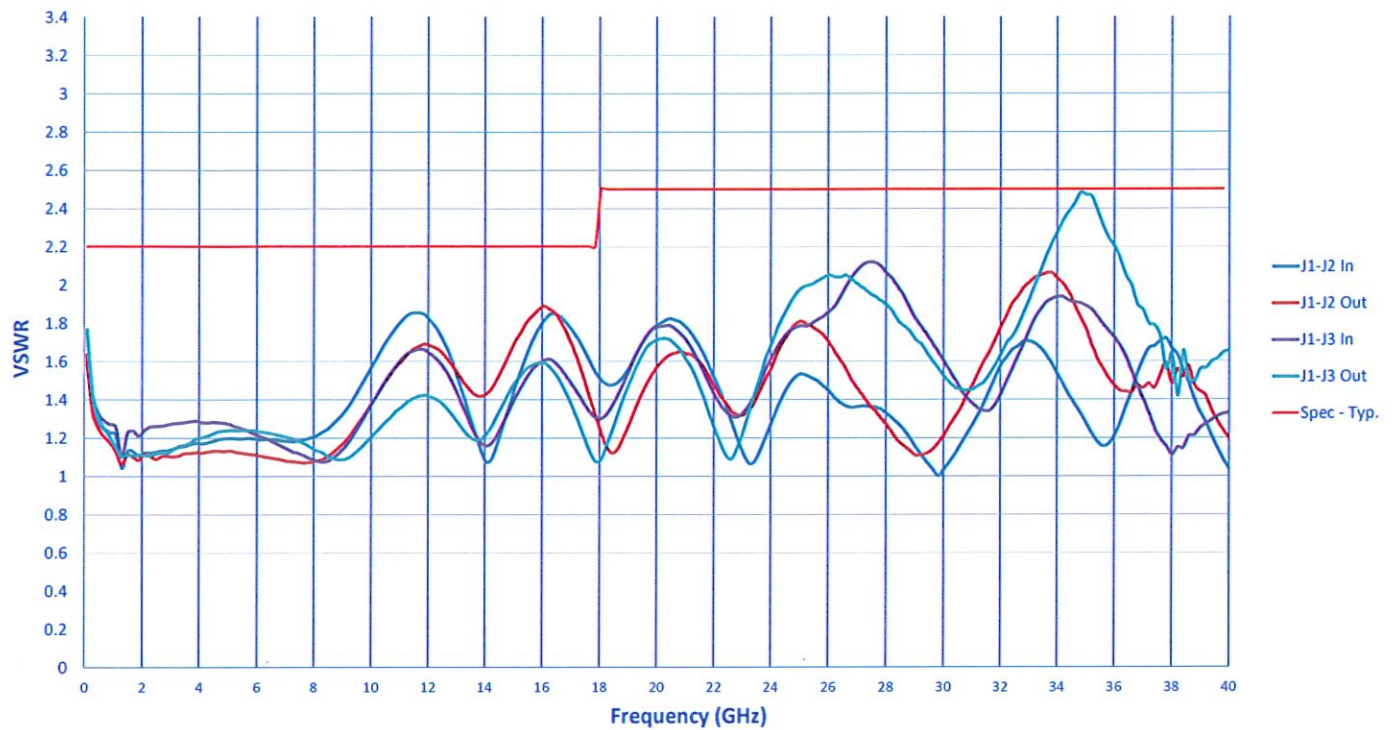
VSWR
