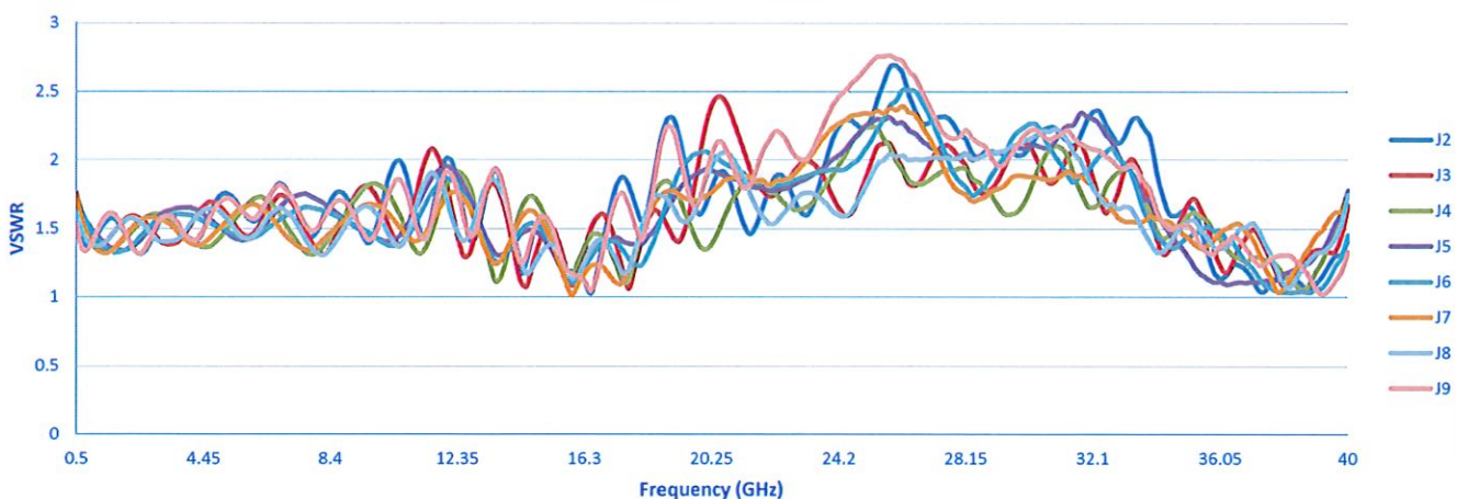
Input VSWR
