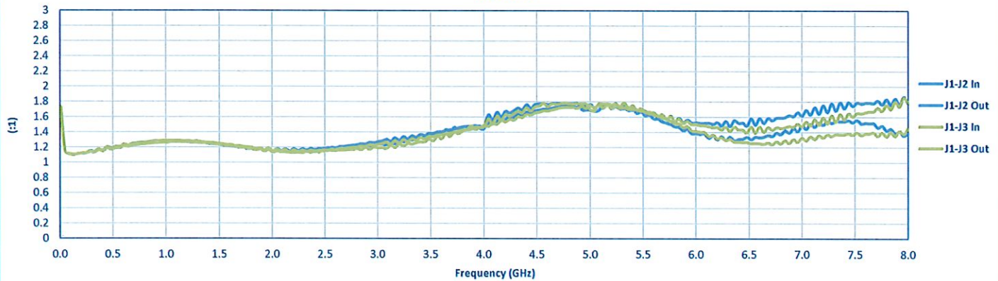
VSWR
