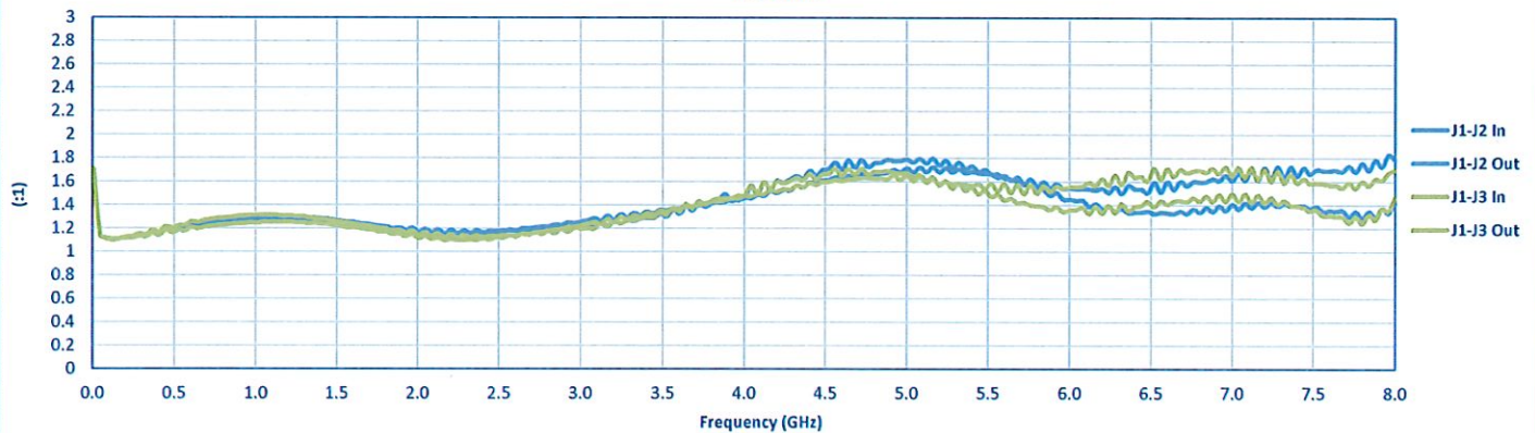
VSWR
