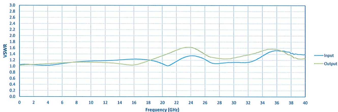
VSWR
