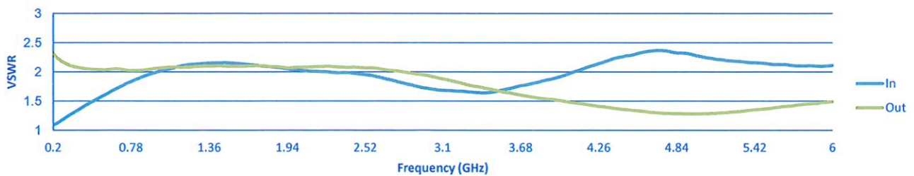
VSWR
