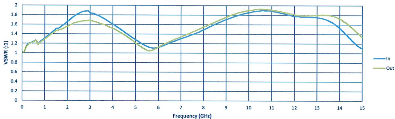
VSWR
