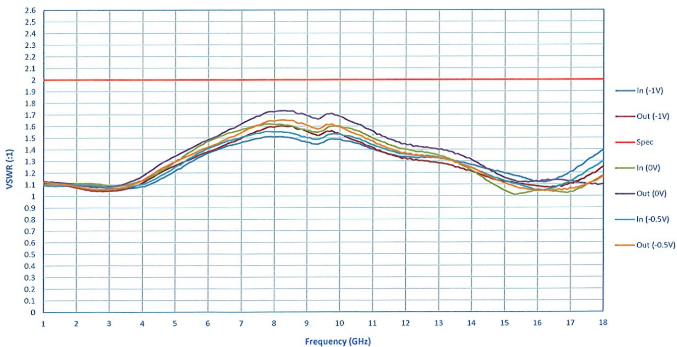
VSWR
