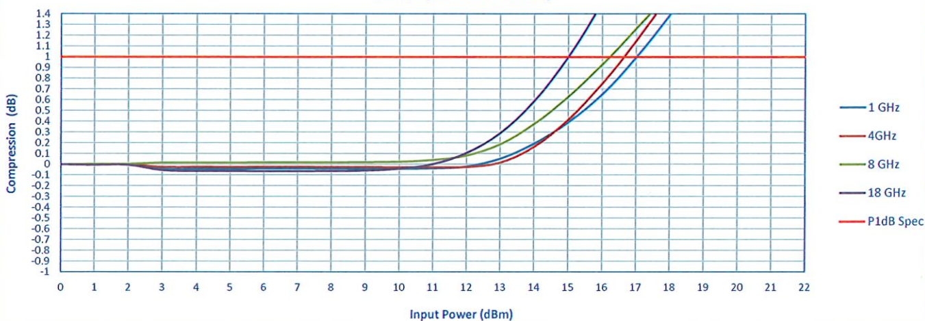
P1dB (-0.5 VDC Bias)
