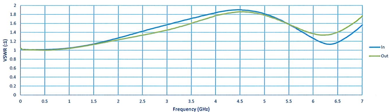
VSWR
