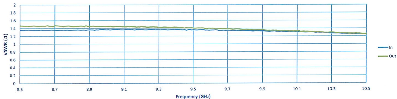
VSWR
