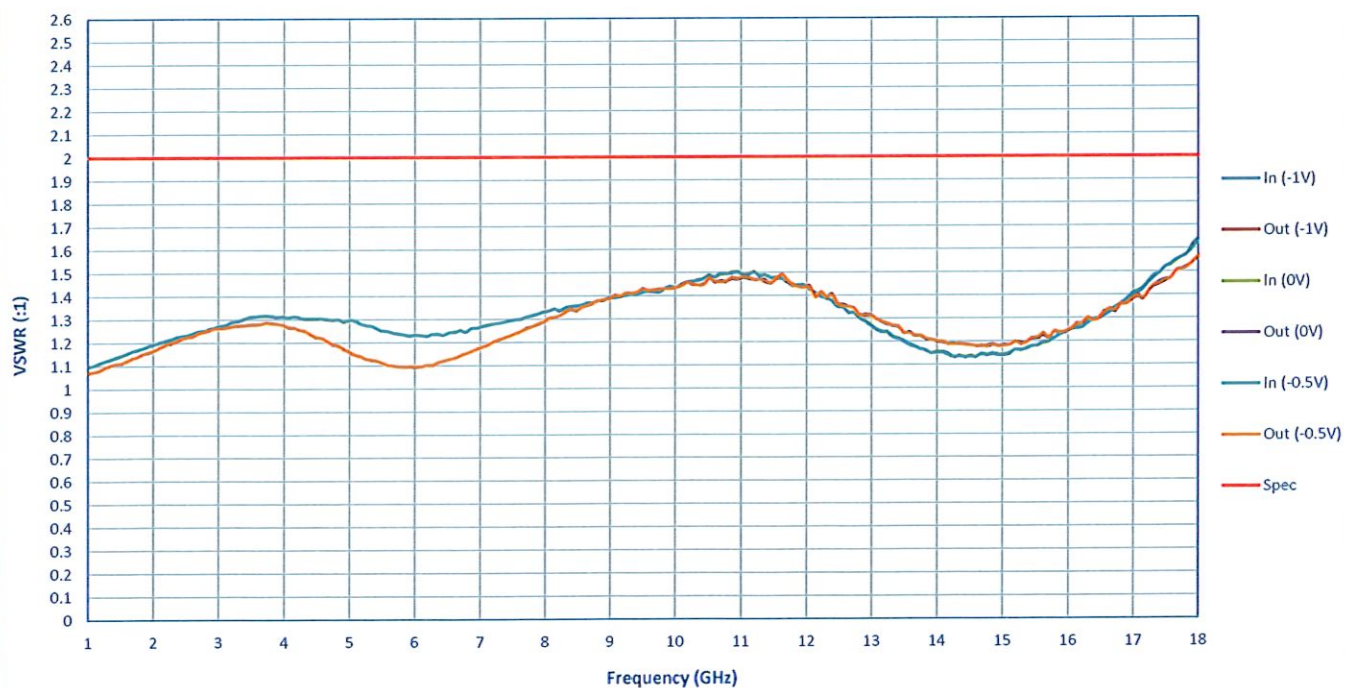
VSWR
