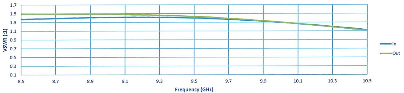
VSWR
