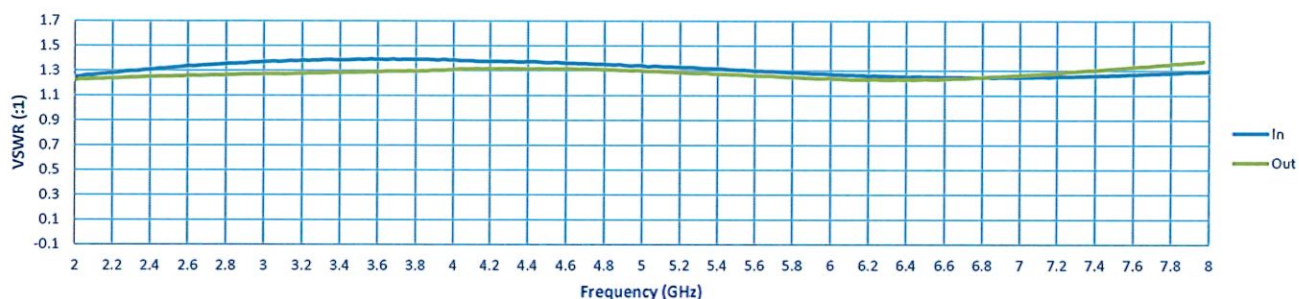
VSWR
