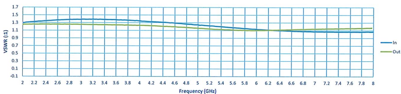
VSWR
