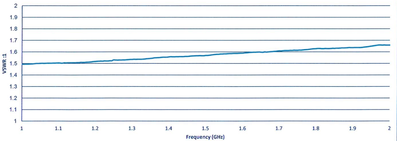
Input VSWR
