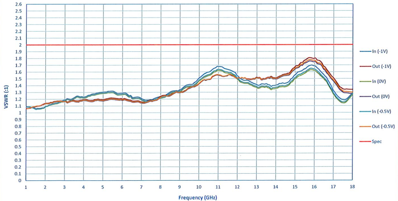
VSWR
