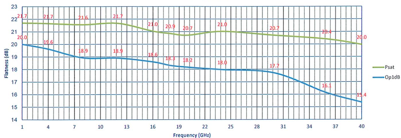
OP1dB & Psat
