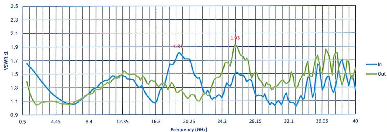
VSWR
