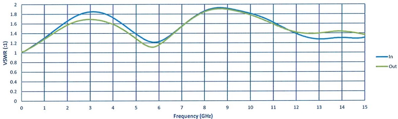
VSWR
