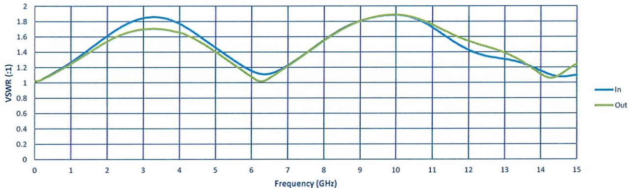
VSWR
