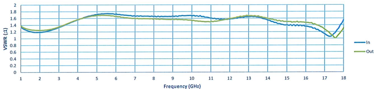
VSWR
