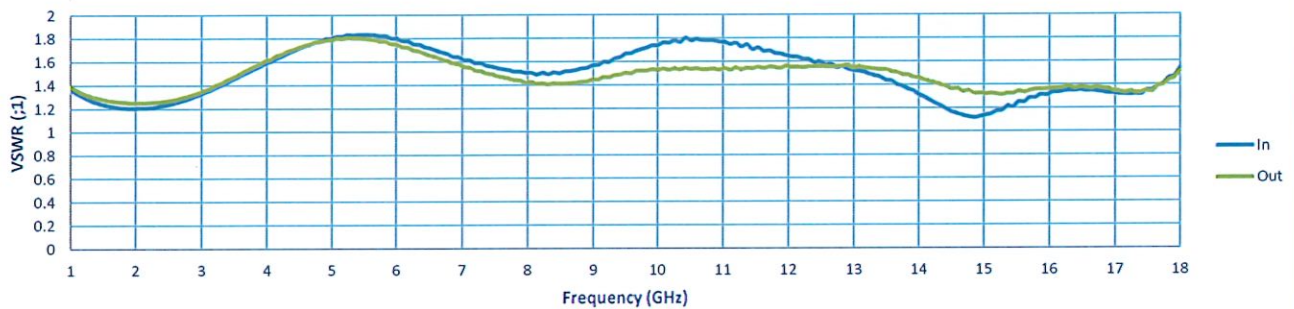
VSWR
