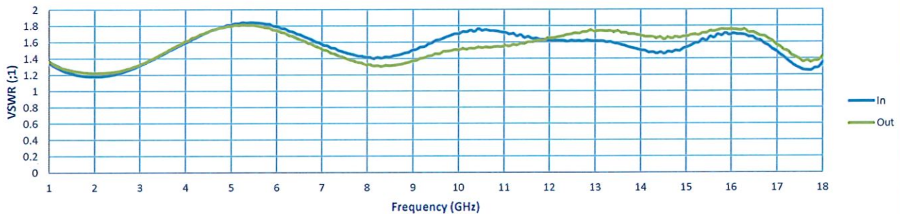
VSWR
