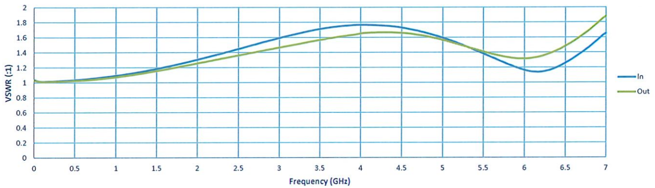
VSWR
