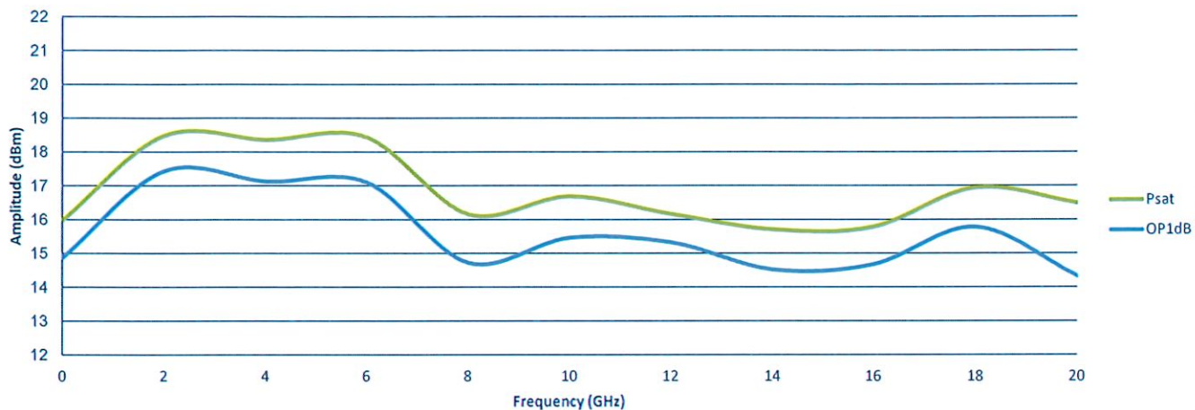
OP1dB & Psat
