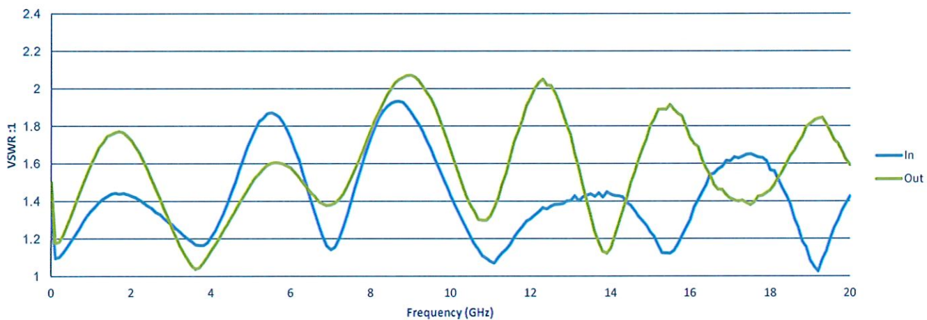
VSWR
