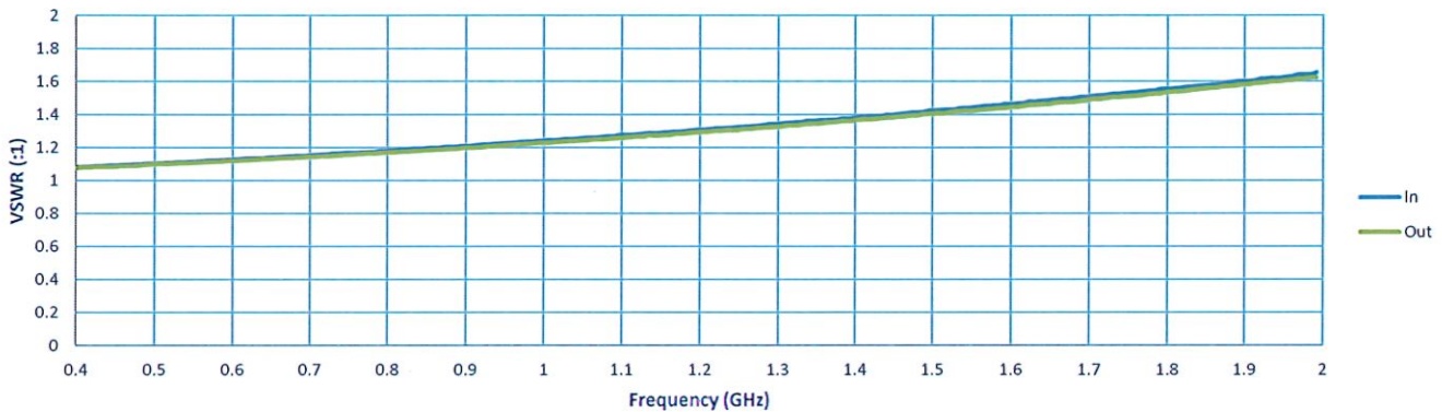
VSWR
