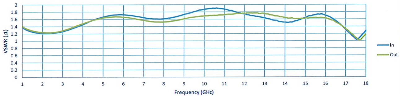
VSWR
