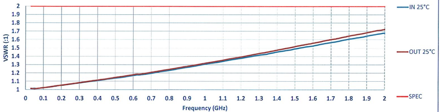
VSWR
