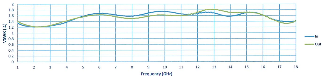
VSWR
